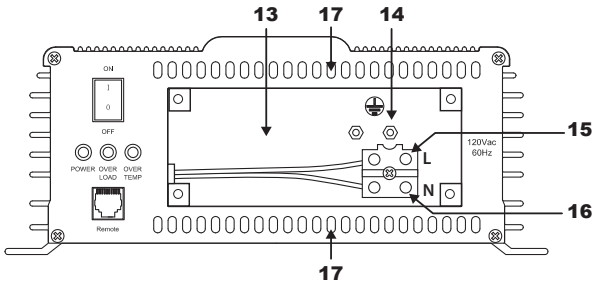
PST-1500 & PST-2000: LE DEVANT - Aperçu du compartiment contenant les bornes de sorties CA pour le câblage.
