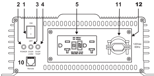
PST-1500 & PST-2000: LE DEVANT
