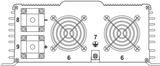
PST-1500 & PST-2000: LA DERRIÈRE
