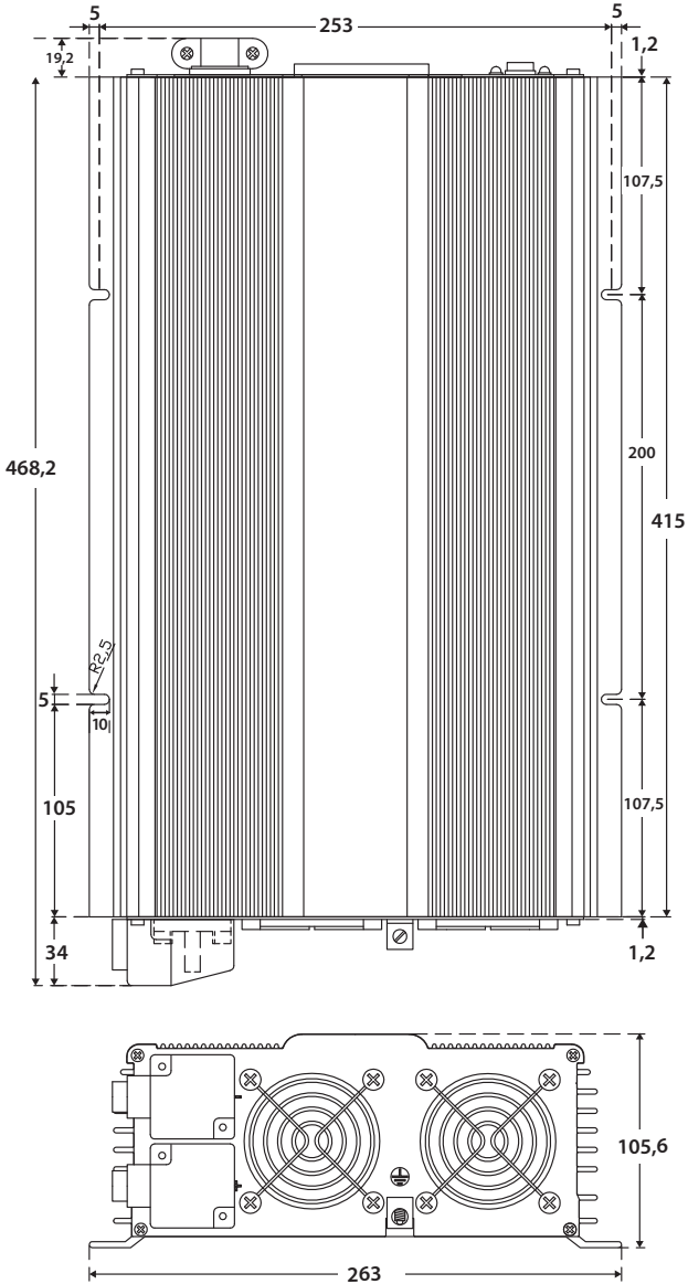
Fig. 8.1: Les Dimensions Générales et Rainures de Montages des PST-1500-12 et PST-1500-24 (NB: Dimensions en mm)
